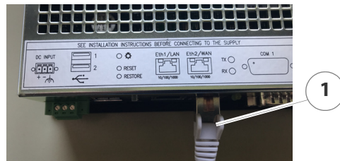
Abbildung 2/2 - Netzwerkanschluss Display HDG Control Pro
