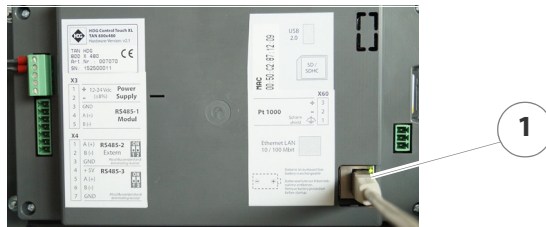
Abbildung 2/1 - Netzwerkanschluss Display HDG Control
